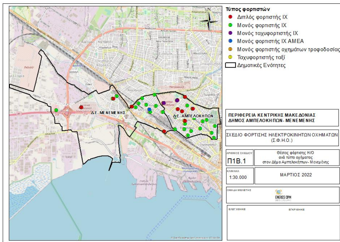
Εικόνα 1: Προτεινόμενες θέσεις φόρτισης Η/Ο στο Δήμο Αμπελοκήπων-Μενεμένης ανά τύπο οχήματος
