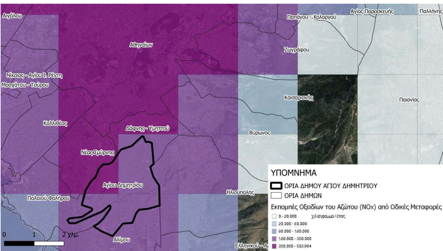
Χάρτης 10. Εκπομπές Οξειδίων του Αζώτου (NOx) από Οδικές Μεταφορές
